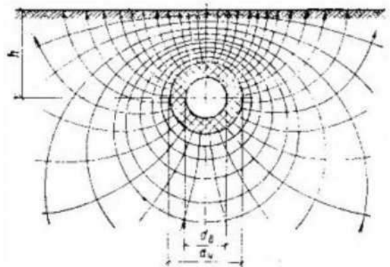
Изолированный трубопровод
